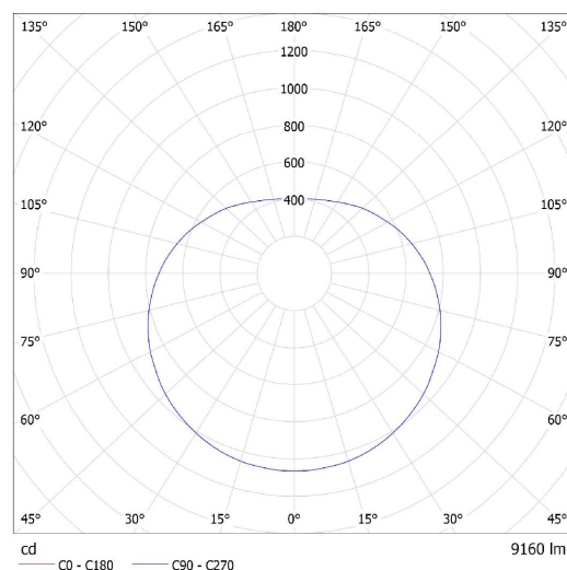
Lucis ZL1.PX1.770 PE DIADEM MAX PE LED / LDC (Polar)
